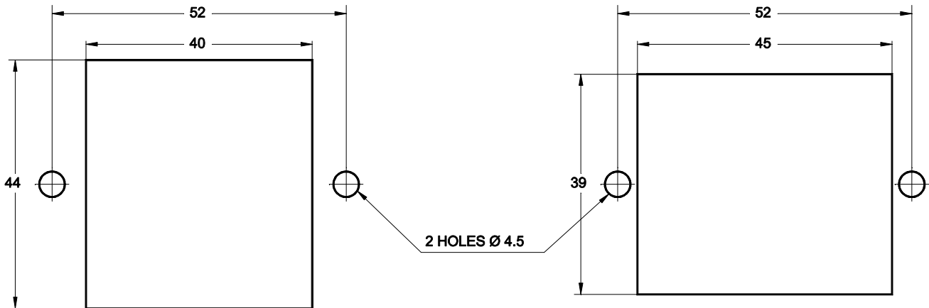
MOUNTING CUT OUT DECOUPE DE LA STRUCTURE
